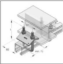
Zacisk jarzmowy – zestaw montażowy M10 45/60
